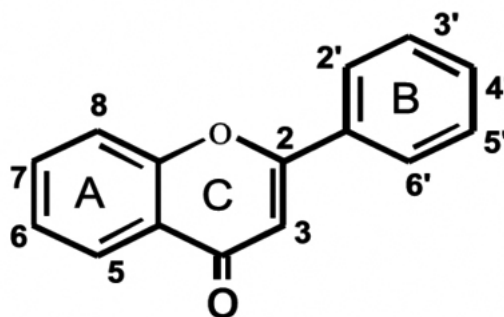
Figura 46. Estructura del anillo pirona donde se representan las sustituciones más frecuentes encontradas en los flavonoides
