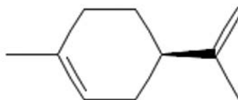
Figura 47. Estructura química del limoneno
