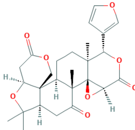
Figura 48. Estructura química básica de los limonoides.
