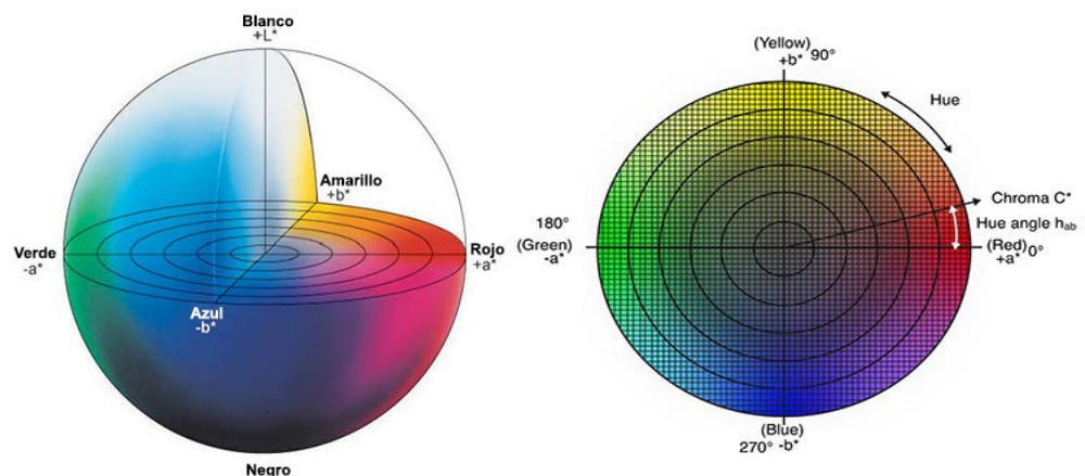
Figuras 34-35. Parámetros de color CIELab. Representación tridimensional de los parámetros cromáticos (izquierda). Coordenadas de color CIELab en el plano (derecha)
